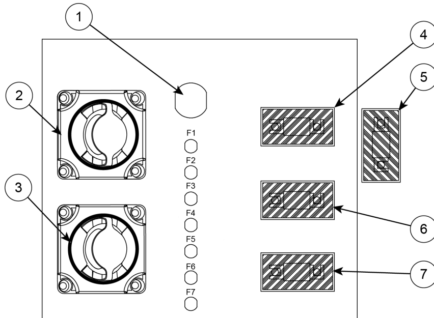
Figur 8.1 Cross 75 BR hovedbryter og sikringspanel
