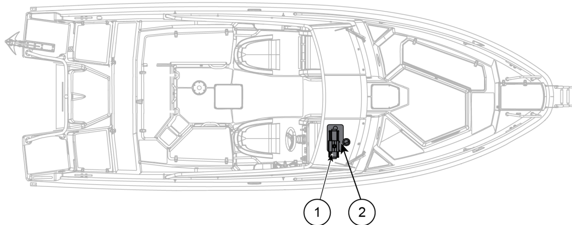
Figur 6.2 Cross 75 BR drivstoffdrevet utstyr
