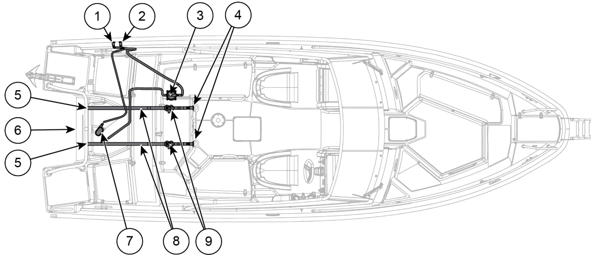
Figur 9.1 Cross 75 BR lensepumper og drenering
