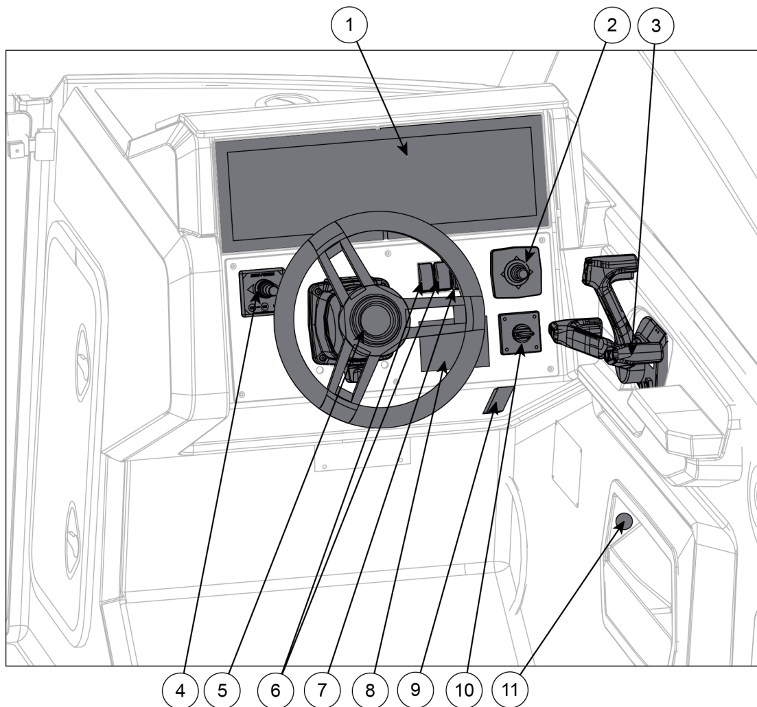
Figur 5.1 Cross 75 BR styrestasjonskontroller
