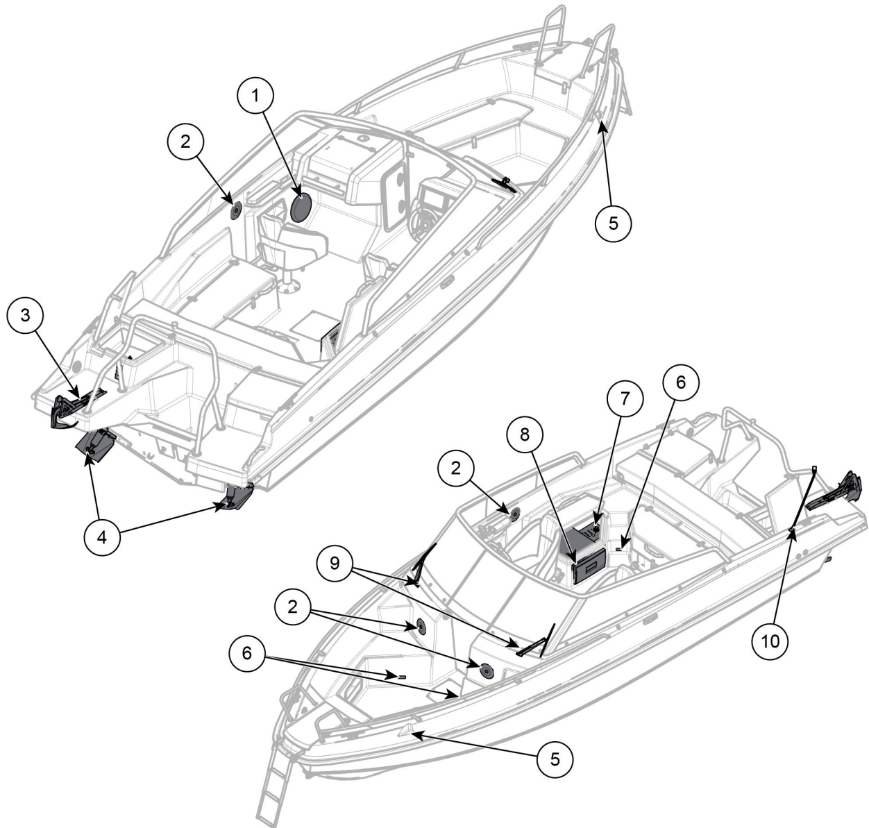
Figur 8.2 Cross 75 BR elektrisk utstyr
